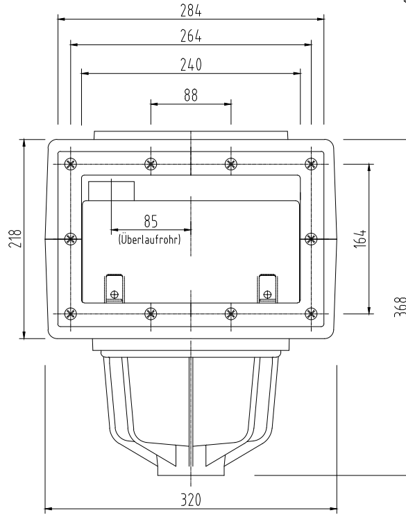
Skimmer mit Kunststoff-Flansch Art.Nr. 152410
